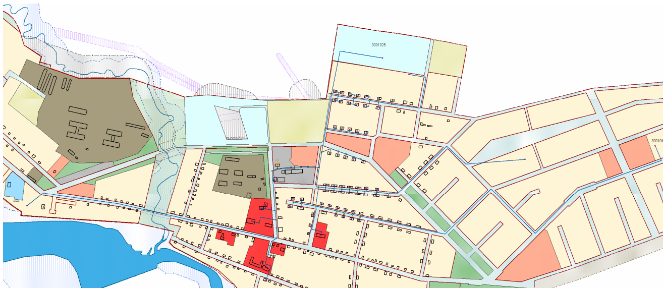
Рисунок 2. Зона действия котельной.
